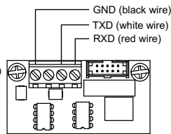
SA-232 wiring
